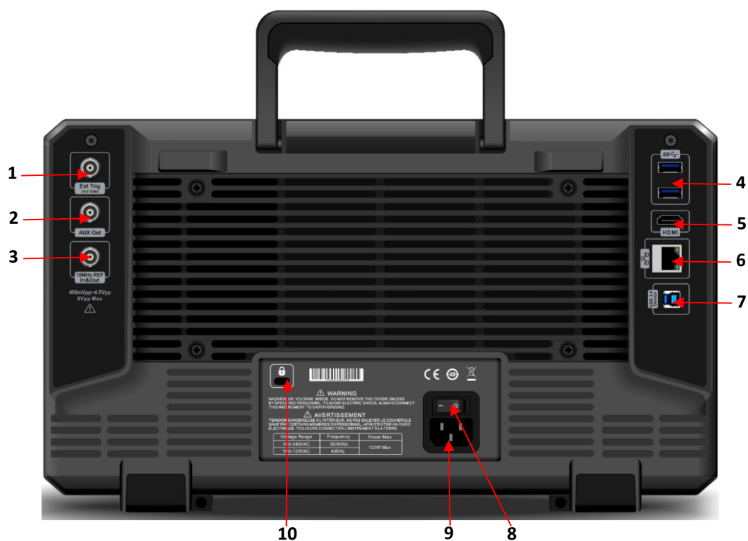
示波器后面板
