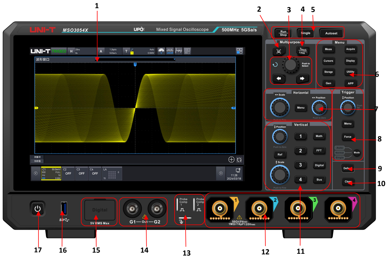
示波器前面板
